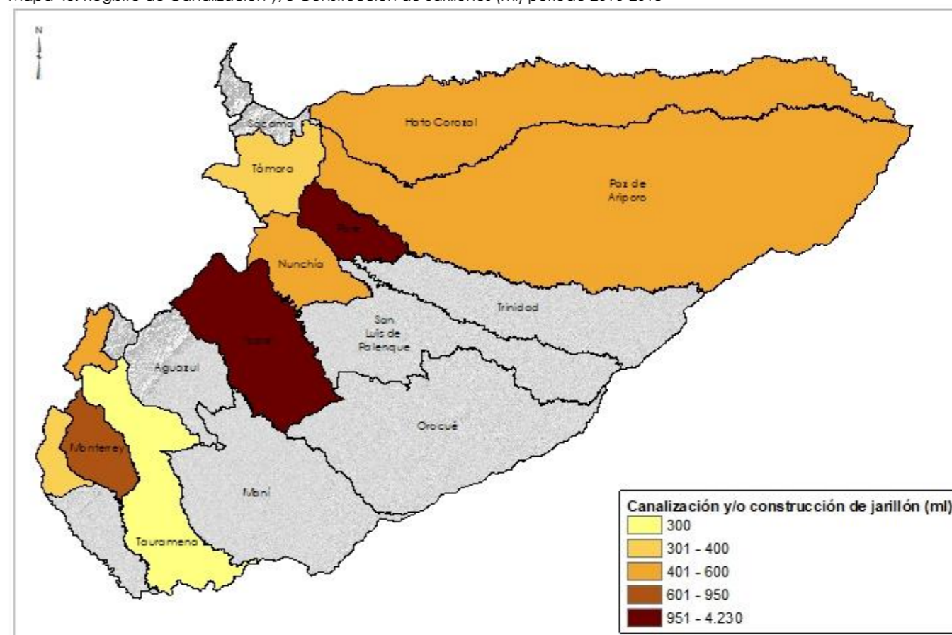
Mapa 45. Registro de Canalización y/o Construcción de Jarillones (ml) periodo 2016-2018
