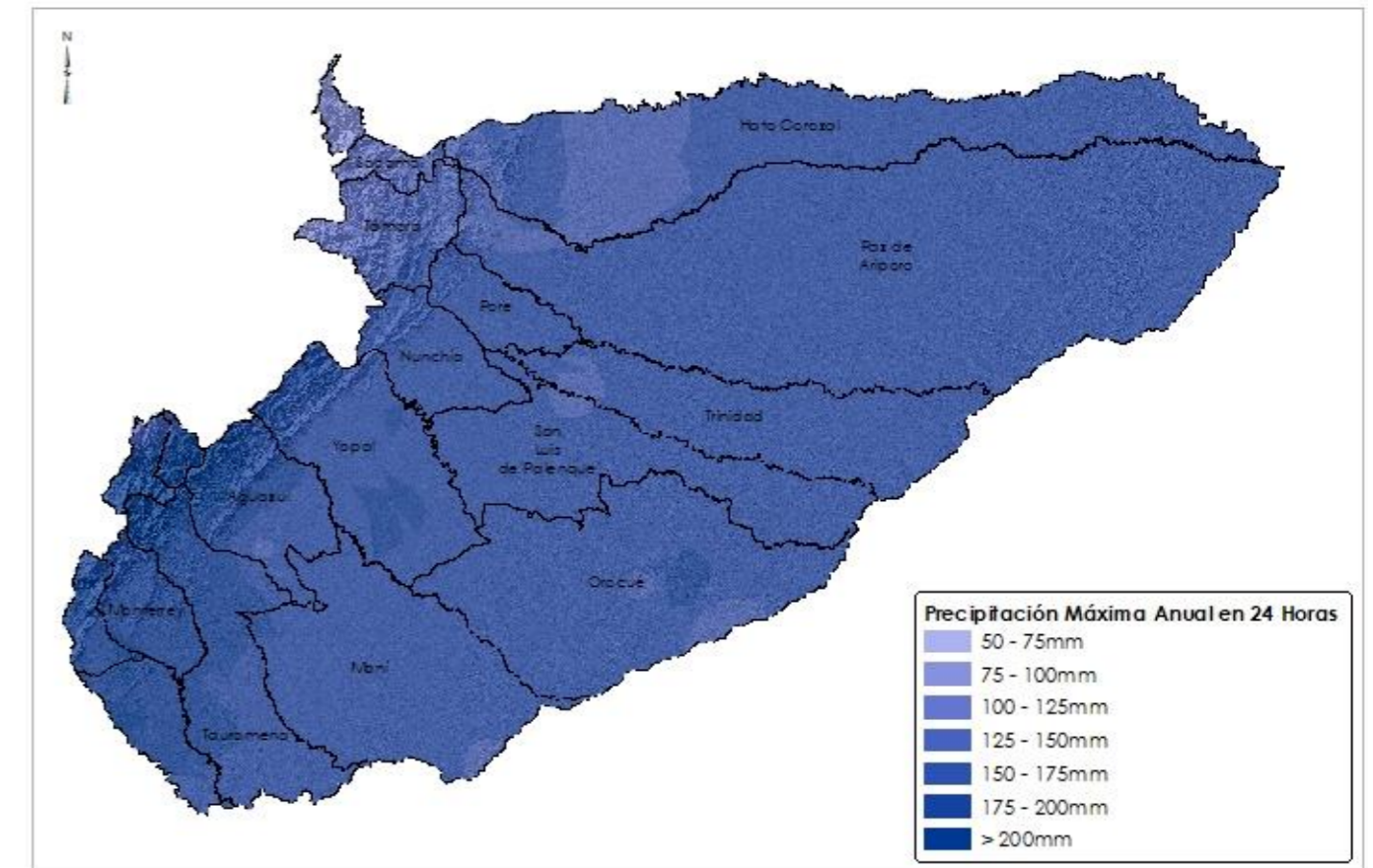
Mapa 26. Precipitación Máxima Anual en 24 horas (mm) Durante el Periodo 1981 – 2010 para el Departamento de Casanare
