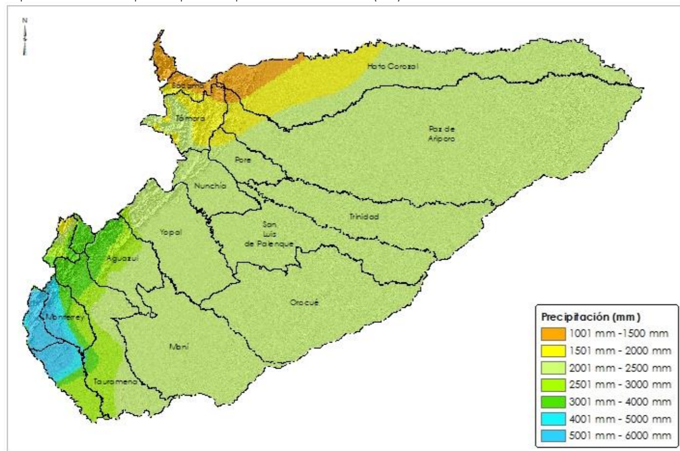
Mapa 29. Escenario Precipitación para el Departamento de Casanare (mm) Periodo 1976-2005
