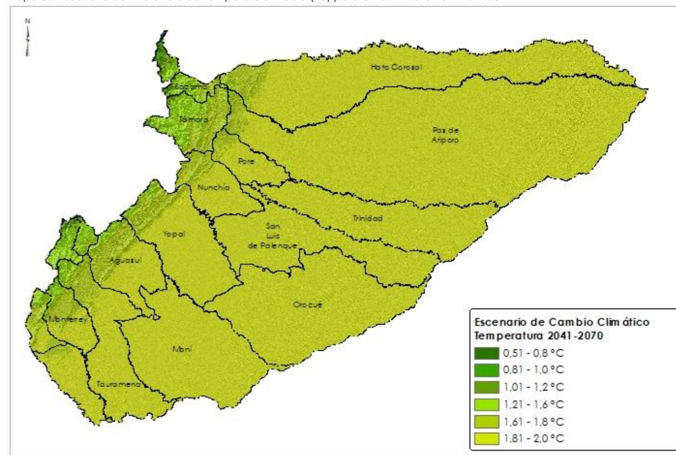
Mapa 35. Escenario de Diferencia de Temperatura Media (°C) para el 2041 - 2070 Vs 1976-2005
