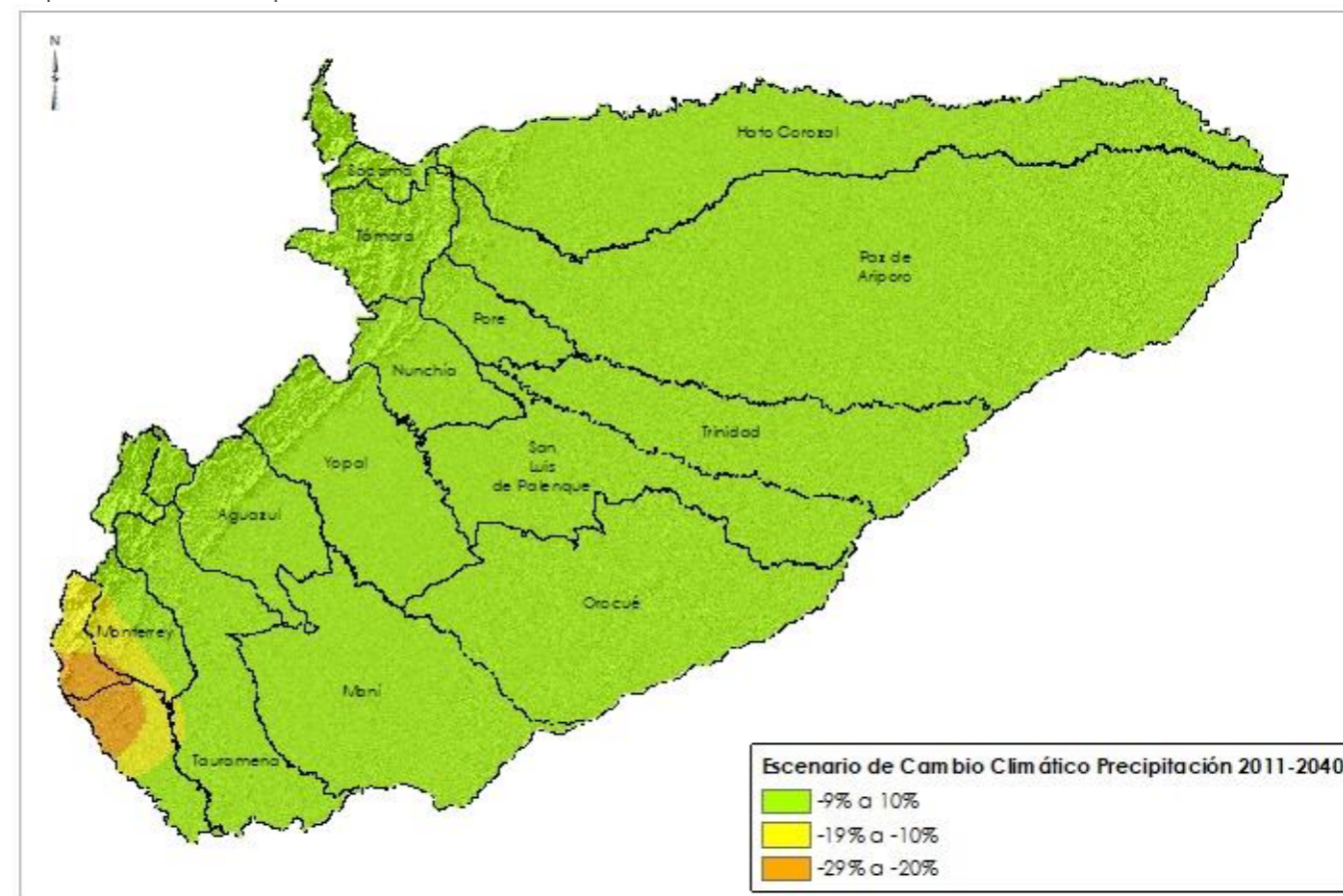
Mapa 30. Escenario Precipitación Ensamble Multiescenario 2011 - 2040 Vs 1976-2005
