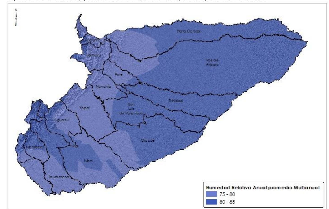
Mapa 28. Humedad Relativa (%) Anual Durante el Periodo 1981 – 2010 para el Departamento de Casanare
