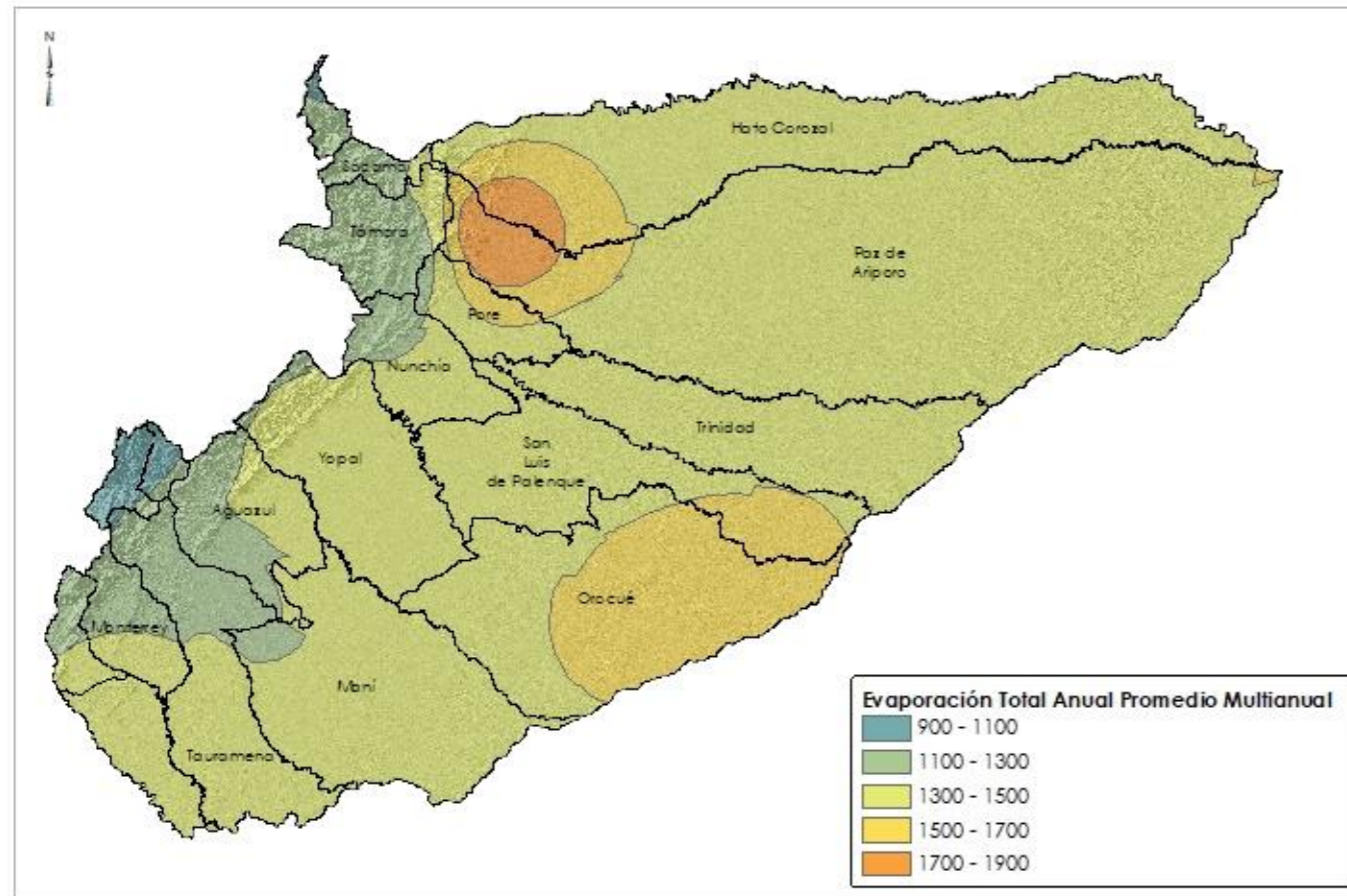
Mapa 27. Evaporación Total Anual Promedio Anual Máxima Anual en 24 horas (mm) Durante el Periodo 1981 – 2010 para el Departamento de Casanare
